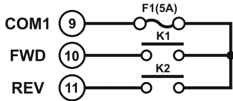
Push button 1~2
